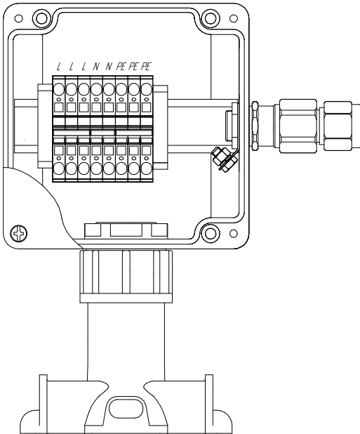
КСТ-КС-П-L(6)/3;N(6)/2;PE(6)/3-П-В: НПС(7,5x5-13,8x6,6)/1-D:БКО(14-22)/1
